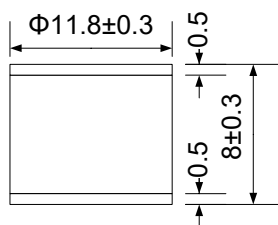
图 1: M0 无引线
