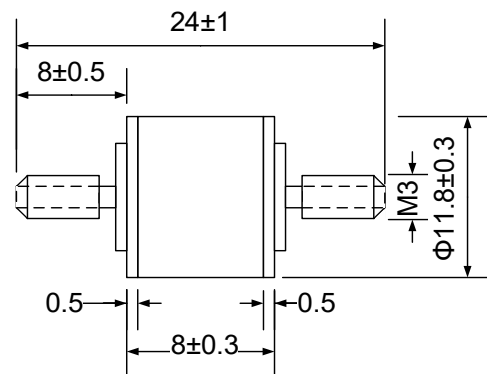
图 3: M3 螺纹型
